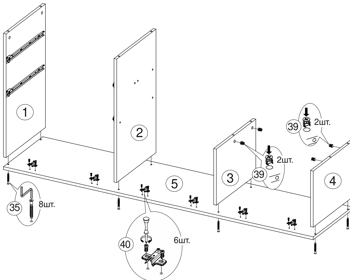
Рис.4 Установка Опор
