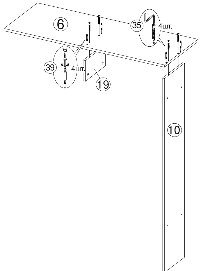
Рис.8 Сборка верхней части гостиной (Крышка тумбы)
