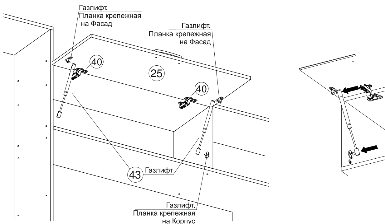
Рис.14 Установка газлифта
